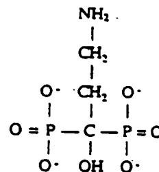
Pamidronate
